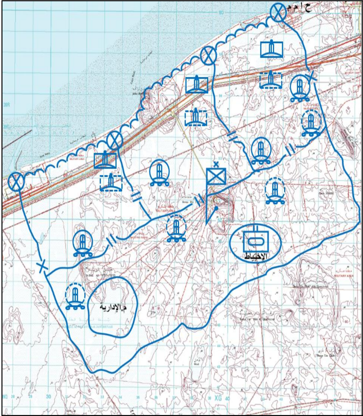
الشكل رقم (6) انفتاح أسلحة الدفاع الجوي عند إسناد مجموعة اللواء في الدفاع الساحلي
